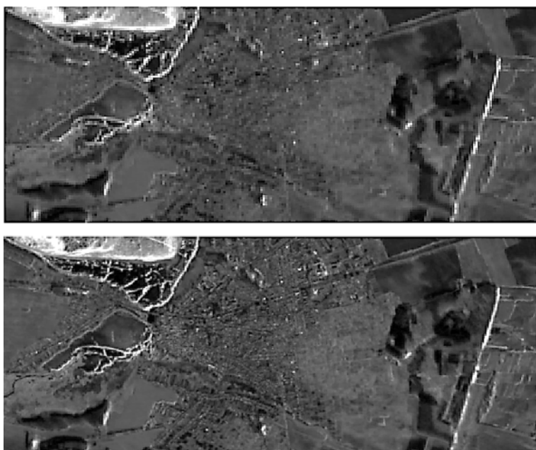
Рис. 4. Реалізація паншарпенінгу
