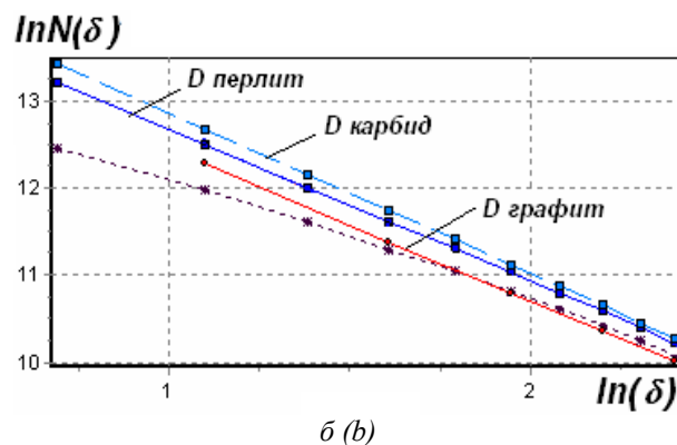
Рис. 2. Реализация расчета фрактальной размерности элементов структуры чугуна марки СПХН: D_{перлит} = 1,759 ; D_{графита} = 1,546 ; D_{карбид} = 1,851 / Fig. 2. Implementation of the calculation of the fractal dimension of the elements of the structure of cast iron СПХН: D_{perlite} = 1,759 ; D_{graphite} = 1,546 ; D_{carbide} = 1,851
