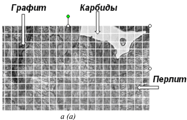
Рис. 2. Реализация расчета фрактальной размерности элементов структуры чугуна марки СПХН: D_{перлит} = 1,759 ; D_{графита} = 1,546 ; D_{карбид} = 1,851 / Fig. 2. Implementation of the calculation of the fractal dimension of the elements of the structure of cast iron СПХН: D_{perlite} = 1,759 ; D_{graphite} = 1,546 ; D_{carbide} = 1,851
