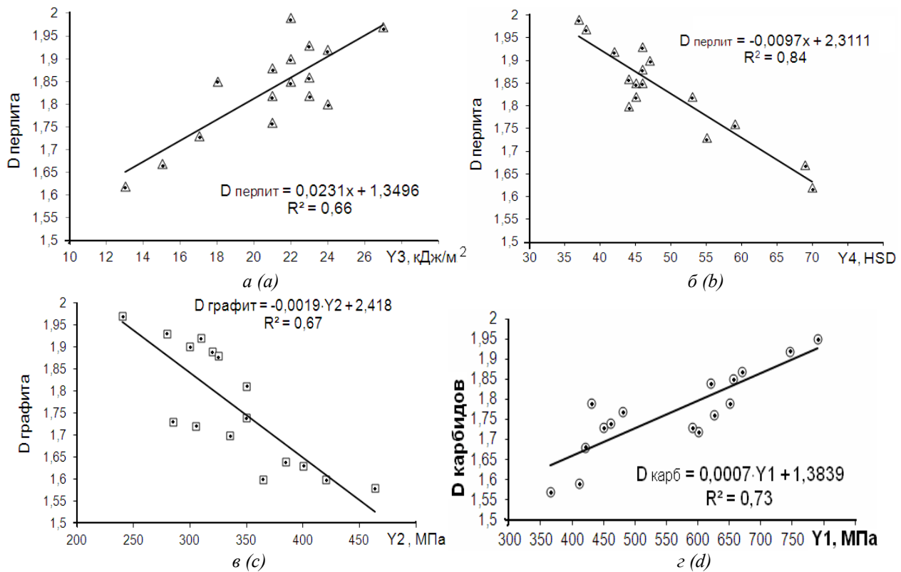
Рис. 3. Соотношения между механическими свойствами чугуна и фрактальными размерностями элементов его структуры: а – КС; б – HSD; в – \sigma_B ; г – \sigma_{изз} / Fig. 3. Relations between the mechanical properties of cast iron and the fractal dimensions of the elements of its structure: a – KC; b – HSD; c – \sigma_B ; d – \sigma_{изз}
