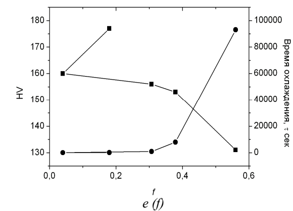
Рис. 3. Зависимость мультифрактальных характеристик перлита (а, в, д) и феррита (б, з, е) от твердости и времени охлаждения образцов / Fig. 3. Dependence of multifractal characteristics of perlite (a, c, e) and ferrite (b, d, f) on the hardness and cooling time of the samples
