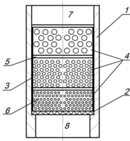
Рис. 2. Будова фільтра для очищення води
