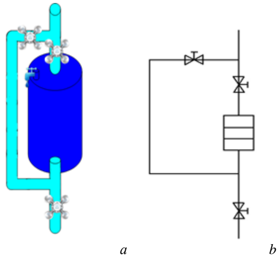
Рис. 1. Зовнішній вигляд фільтра для очистки води (а) та схема (б) його врізання у водопровідну мережу.
