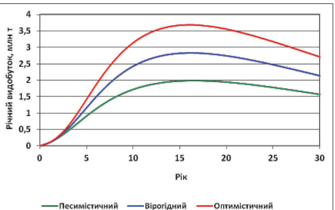
Рис. 6. Сценарії видобутку від залучення у розробку залишкових запасів нафти
