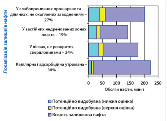
Рис. 4. Середньостатистичний розподіл залишкової нафти і потенціал її залучення до розробки
