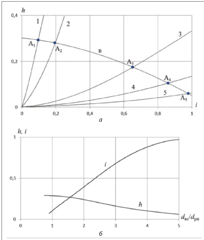
Рис. 3. Визначення режиму роботи ежекційної системи пристрою для промивання піскових корків: a – визначення робочих точок струминного насоса для різних співвідношень діаметрів всмоктувального патрубку та робочої насадки: 1 – \frac{d_{vc}}{d_{рн}}=1 ; 2 – \frac{d_{vc}}{d_{рн}}=1,414 ; 3 – \frac{d_{vc}}{d_{рн}}=3 ; 4 – \frac{d_{vc}}{d_{рн}}=4 ; 5 – \frac{d_{vc}}{d_{рн}}=5 ; b – залежність коефіцієнта інжекції i та відносного напору струминного насоса від співвідношення діаметрів \frac{d_{vc}}{d_{рн}}
