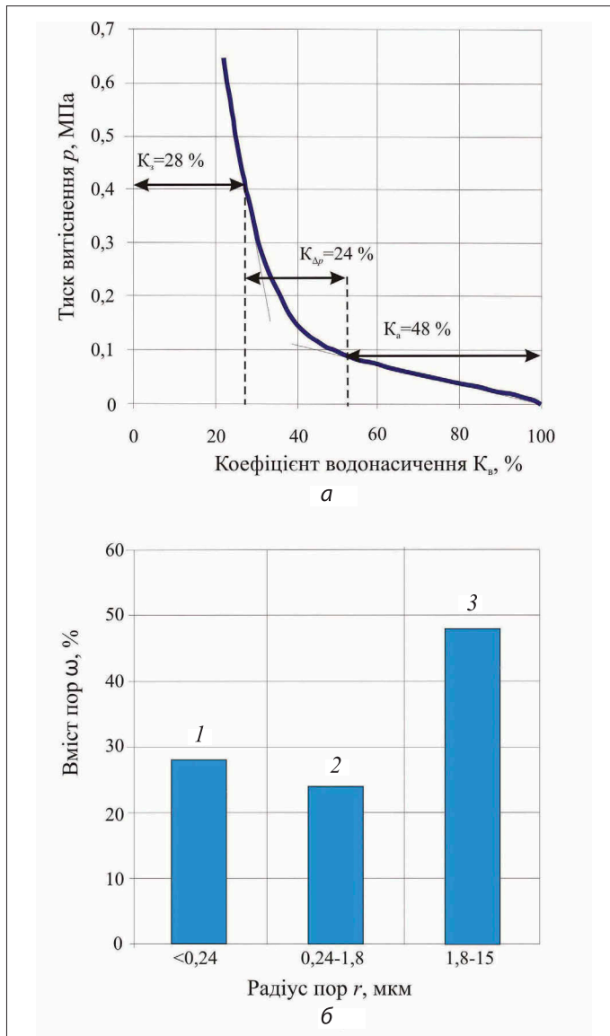
Рис. 1. Крива капілярного тиску (а) і вміст пор різного радіуса (б) для стандартного зразка відкритої пористості 201-46; пори: 1 – субкапілярні; 2 – капілярні; 3 – надкапілярні
