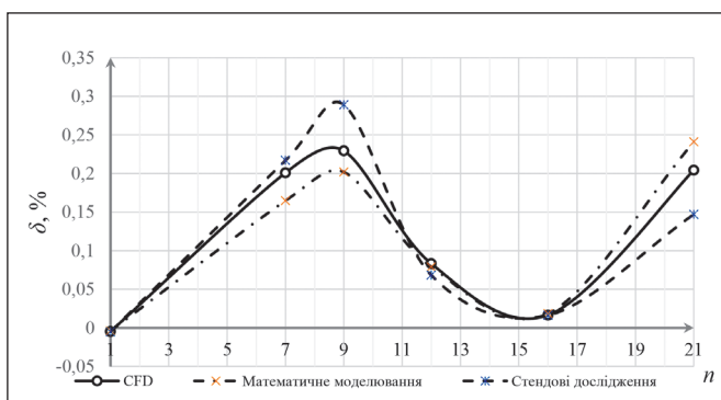
Рис. 3. Похибка приладу на різних відстанях після коліна з поворотом на кут \pi/2 рад
