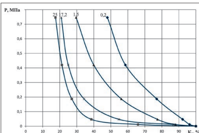
Рис. 4. Порівняльна залежність залишкового водонасичення порід із різними фільтраційними властивостями (шифр кривих – газопроникність у мД)
