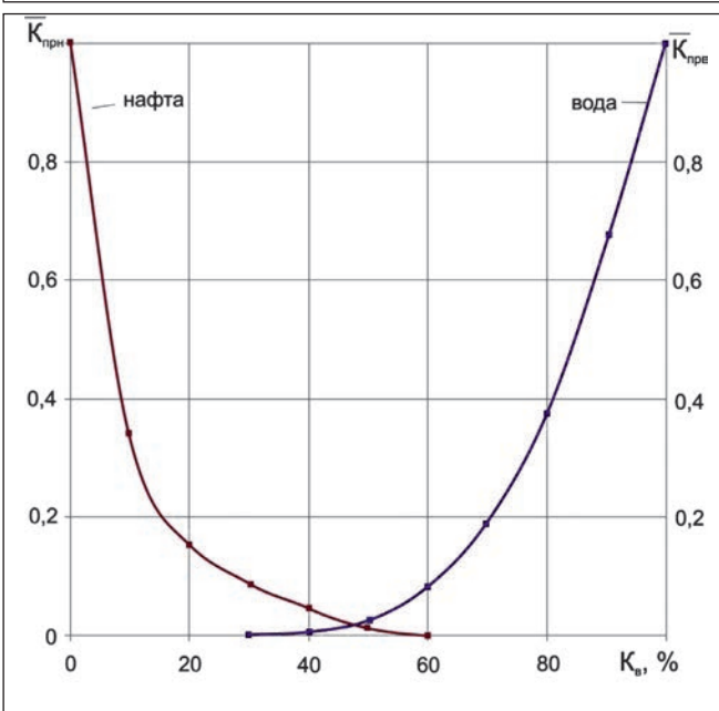
Рис. 5. Залежність відносних фазових проникностей для нафти і води від водонасичення (зразок із K_{\text{гп}}=17,2 мД, K_{\text{н}}=18,8\% , K_{\text{в}}=75\% )
