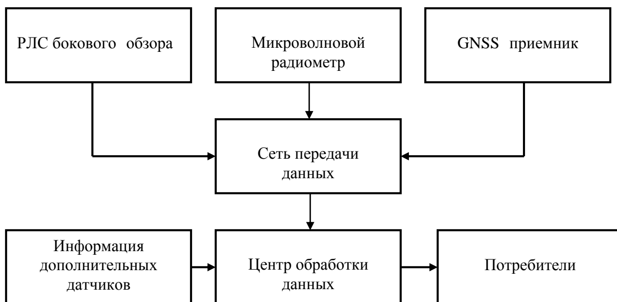
Рис.1. Структурная схема комплекса мониторинга загрязнения водной поверхности
