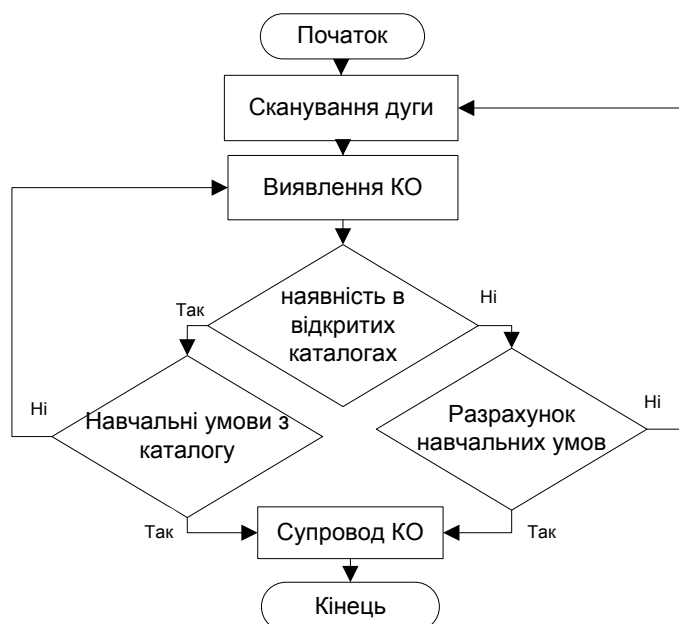
Рис.5. Алгоритм методики ведення зонального каталогу геостаціонарних космічних об'єктів
