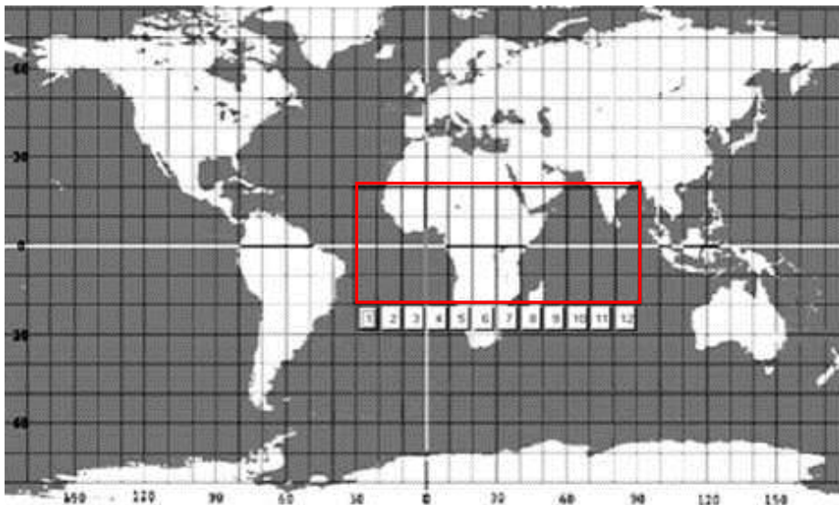
Рис. 3. Дуга геостаціонарної орбіти, яка спостерігається квантово-оптичними системами «Сажень-С»
