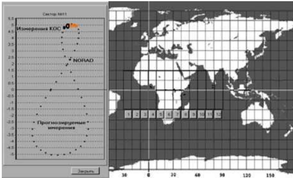
Рис. 8. Идентификация измерений квантово-оптической системы з відкритим каталогом
