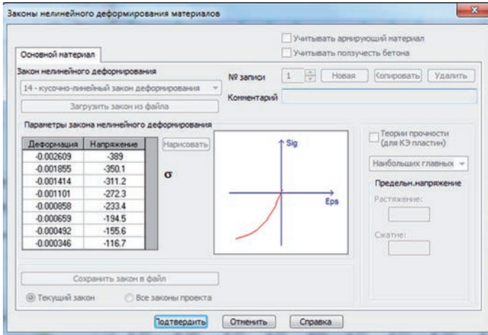
Рис.4. Закон нелінійного деформування для СЕ кладки в моделі.
