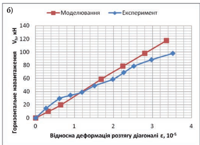
Рис.6. Графіки деформування основних діагоналей зразку БС-БТ та його моделі під дією горизонтальної сили V_{hr} : а – діагональ, що стискається; б – діагональ, що розтягується.
