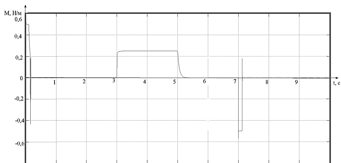
Рис. 7. Переходная функция по моменту
