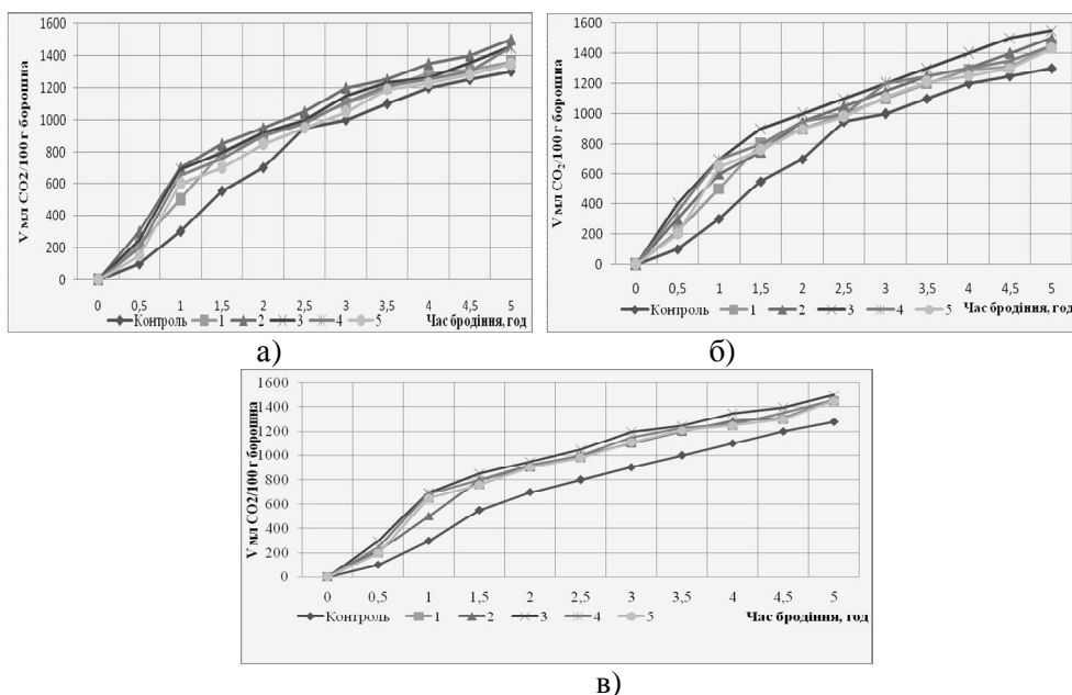
Рис. 1. Динаміка газоутворення при додаванні продуктів переробки хеномелесу:
