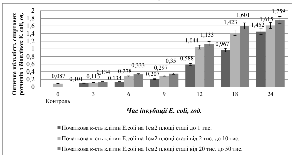
Рис. 2. Формування біоплівки E. coli на нержавіючій сталі марки AISI 321 шорсткістю R_a = 0,63 мкм при температурі 37 °С
