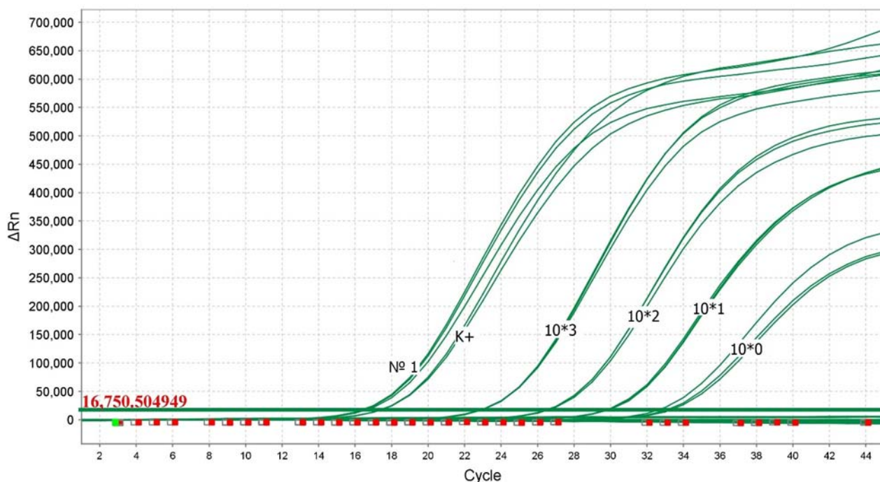
Рис. 2. Криві ампліфікації цільової послідовності вірусу КЧС за ROX: K+ – позитивний контроль; № 1 – РНК вірусу КЧС, штам «Вашингтон»; 10*3, 10*2, 10*1, 10*0 – 10-кратні розведення кДНК вірусу КЧС
