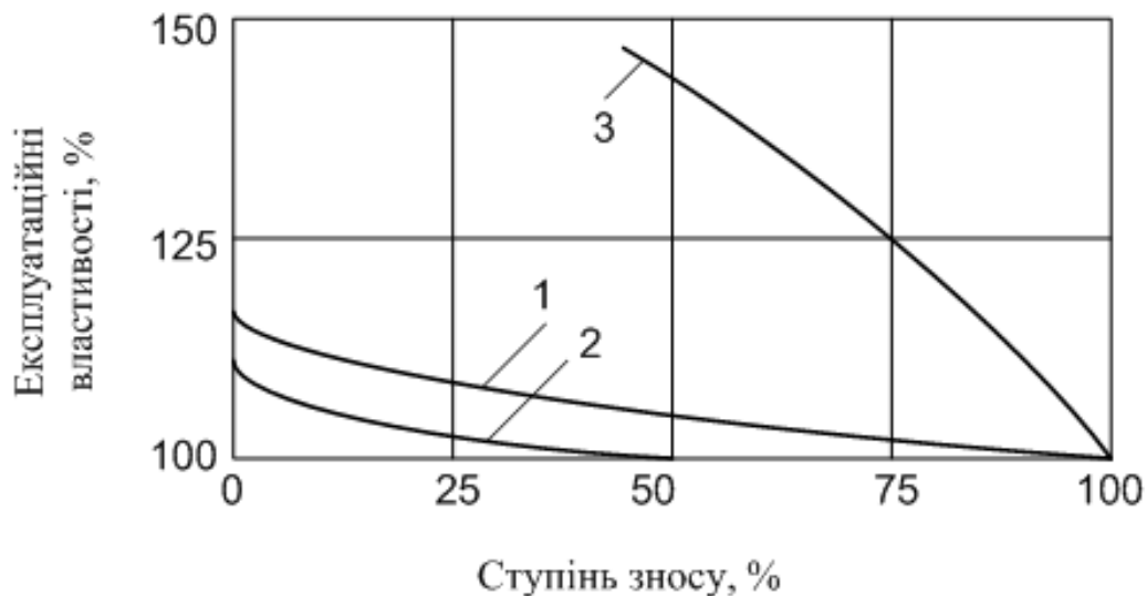
Рис. 1. Зміна експлуатаційних властивостей автомобіля при зношенні протектора: 1 – витрати палива; 2 – час розгону; 3 – сила тяги.
