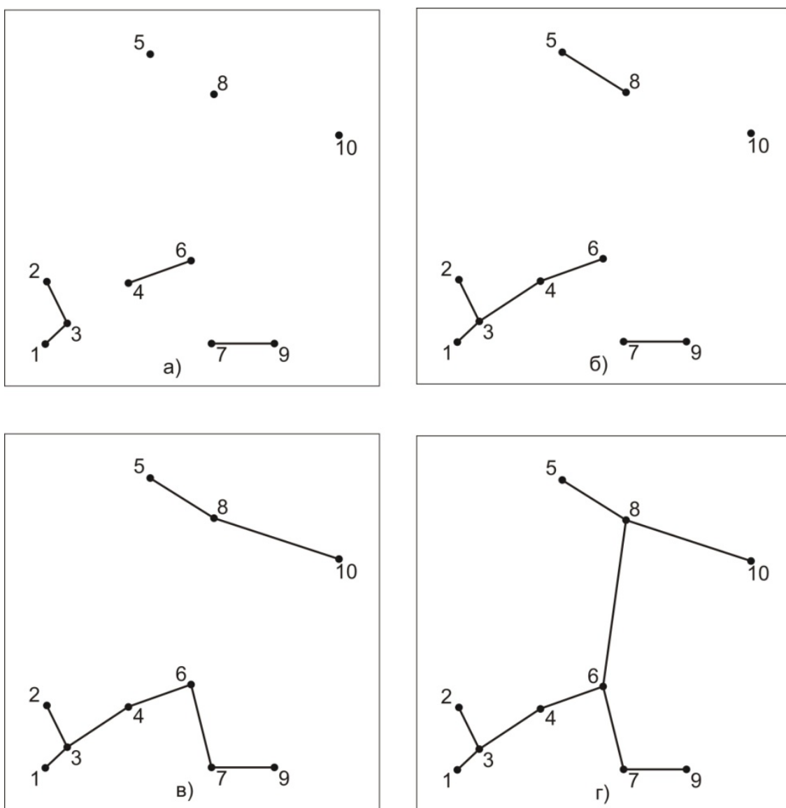
Рис.3. Связывание электропотребителей в единую сеть с наименьшей протяженностью линий при выполнении алгоритма Краскала
