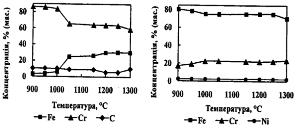
Рис. 2. Середній склад карбідів (а) і зерен матриці (б) в спеченому при різних температурах зразку карбідосталі X17H2-15% об. Cr 3 C 2 .
