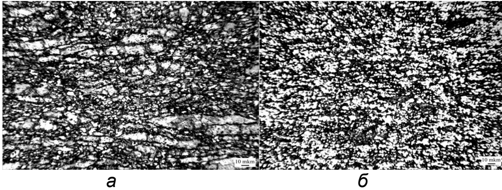
Рис. 1. Мікроструктура гарячештапованих при 1200°C карбідосталей X17H2–7,5% об. Cr 3 C 2 (а), 30% об. Cr 3 C 2 (б), відпалених при 1150°C.
