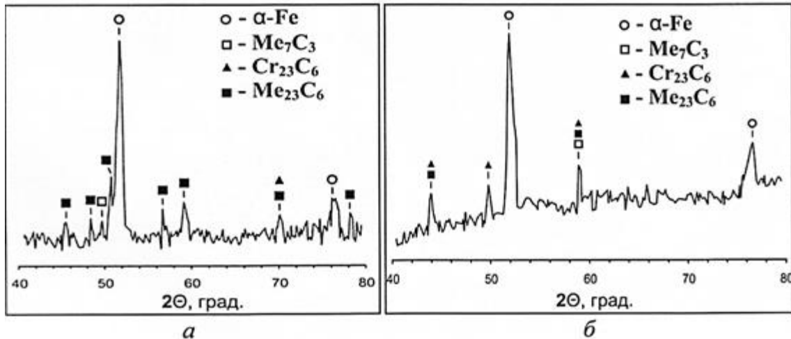
Рис. 3. Дифрактограма карбідосталей X17H2 об. 15% \text{Cr}_3\text{C}_3 , (а) та X13M2 – 15% об. \text{Cr}_3\text{C}_2 (б), спечених при температурі 1250 °С.
