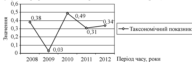
Рис. Динаміка таксономічного показника розвитку підприємства
