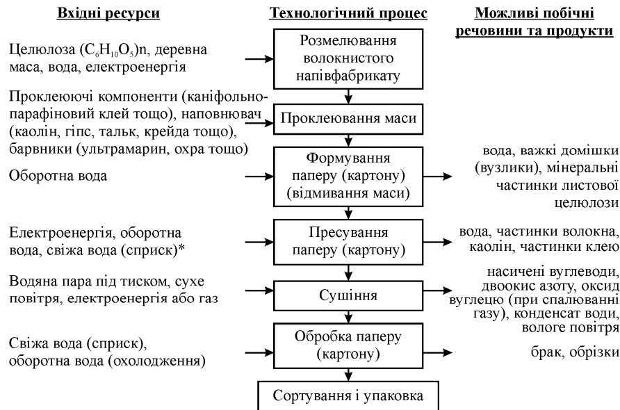
Рис. 2. Загальна схема технологічного процесу виробництва паперу (картону) та його потенційного впливу на довкілля [4]
