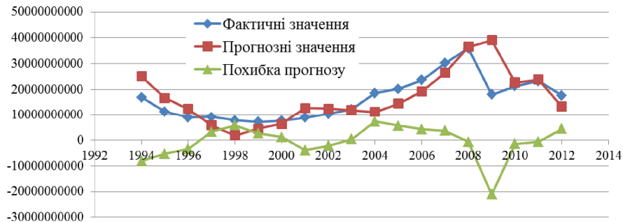
Рис. 7. Прогнозні значення показника внутрішніх валових заощаджень України за допомогою побудованої ARIMA(1, 1, 4)-моделі
