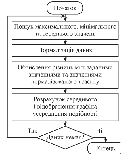
Рис. 1. Блок-схема алгоритму роботи розробленого програмного комплексу прогнозування трафіку потоку в сегменті комп'ютерної мережі
