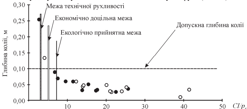
Рис. 2. Залежність глибини колії від індексу рушія за EcoWood проєктом
