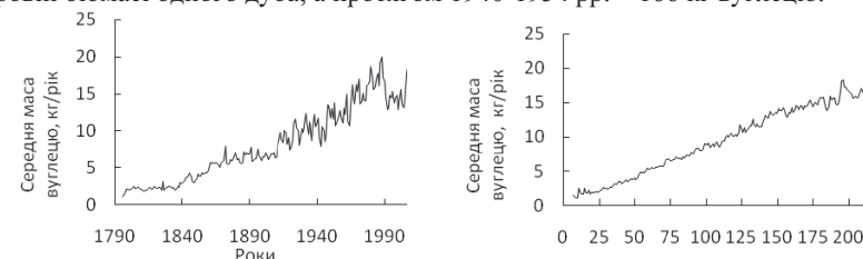
Рис. 2. Щорічна динаміка нагромадження вуглецю у стовбуровій біомасі Q. robur ППСМ "Феофанія"
