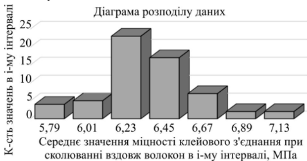
Рис. 6. Гістограма розподілу експериментальних даних міцності клейового з'єднання термодеревини ясеня, обробленої за температурі 220°C упродовж 4-х год, при сколюванні вздовж волокон
