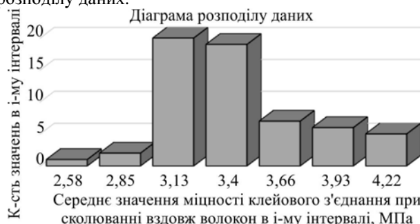
Рис. 5. Гістограма розподілу експериментальних даних міцності клейового з'єднання термодревини ясена, обробленої за температури 160°C упродовж 4-х год, при сколюванні вздовж волокон
