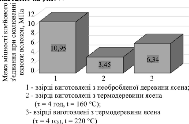
Рис. 7. Результати експериментального дослідження межі міцності клейового з'єднання при сколюванні вздовж волокон
