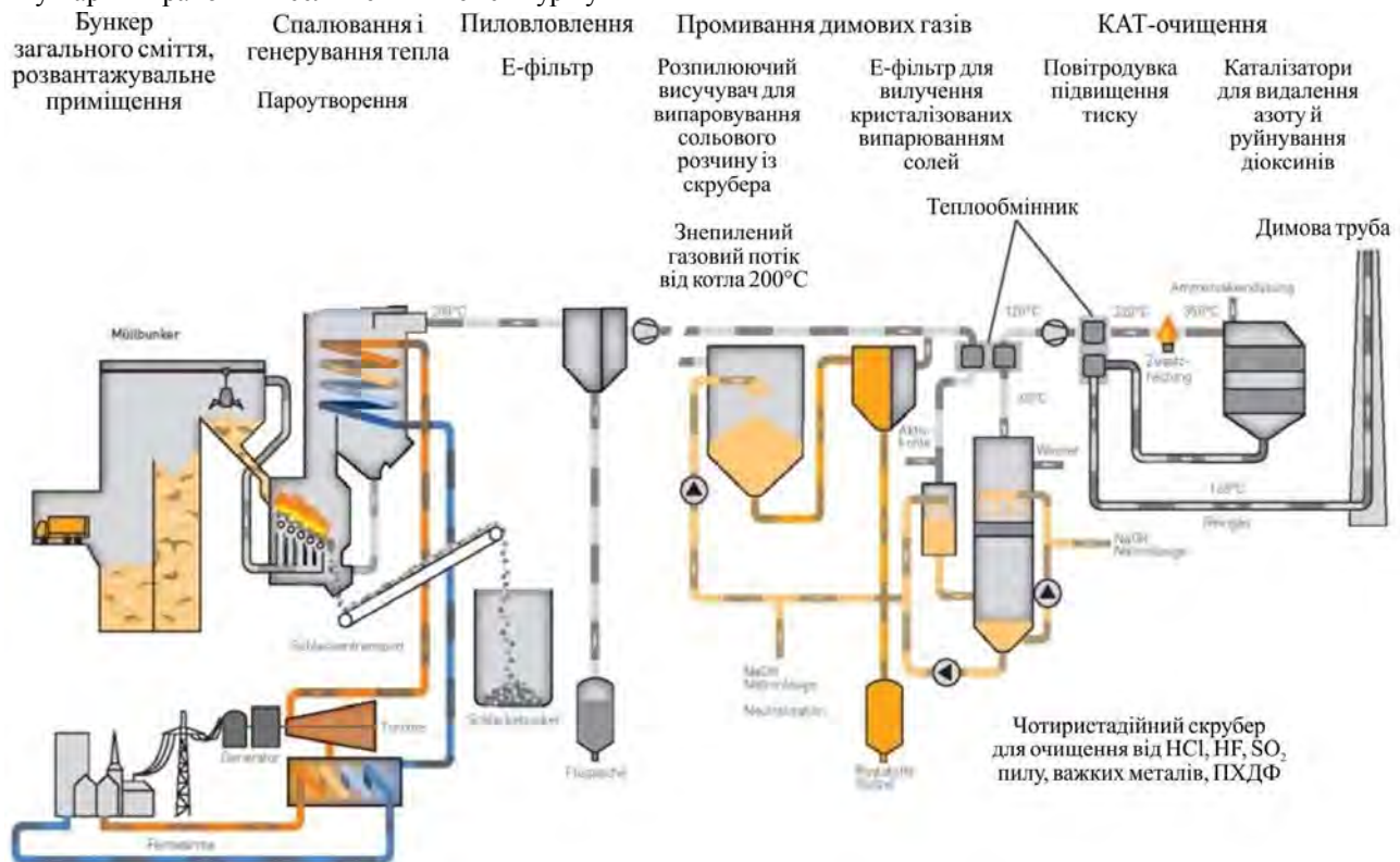
Рисунок. Функціональна схема сміттєспалювального підприємства (Primärenergie veredeln, 2010)
