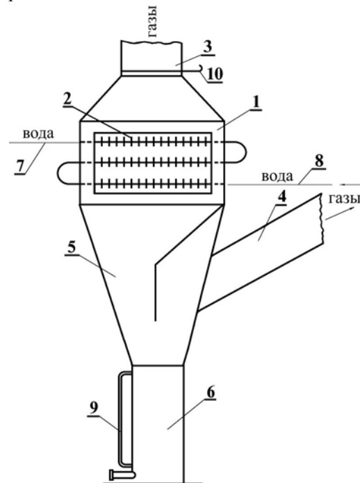
Рис. 1. Модель конденсационного теплоутилизатора
