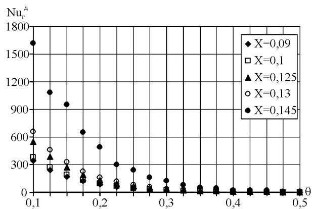
Рис. 6. Зависимость Nu_r^a от температуры \theta при X = 0,09 \div 0,145 кг/кг с.г. и Re_r = 10000
