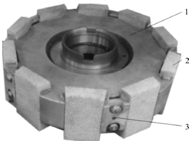
Рис. 1. Шліфувальний круг зі вставними сегментами: 1) корпус; 2) абразивний сегмент (брусочок); 3) затискач
