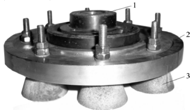
Рис. 2. Багаточашковий абразивний інструмент: 1) фланець; 2) корпус; 3) абразивна чашка
