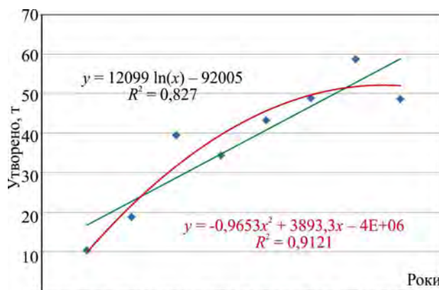
Рис. 5. Регресійні залежності обсягу спалених відходів у Львівській області для отримання енергії
