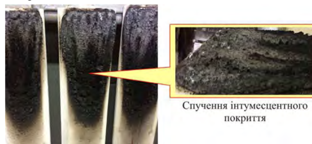
Рис. 5. Результати випробувань модельного зразка, обробленого вогнезахисним інтумесцентним покриттям
