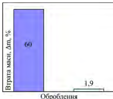
Рис. 3. Результати втрати маси зразків \Delta m , % деревини: 1) необроблена; 2) вогнезахиснена інтумесцентним покриттям на основі органічних і мінеральних речовин
