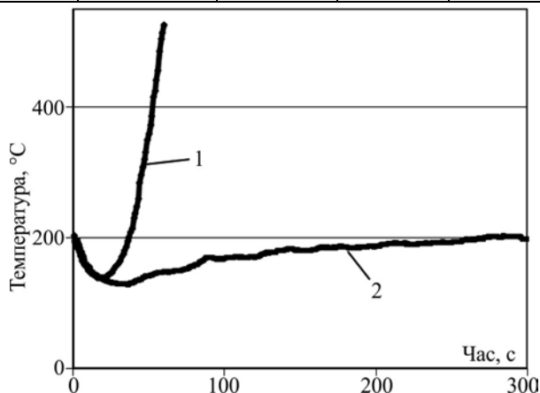
Рис. 2. Динаміка наростання температури димових газів під час випробувань деревини: 1) необроблена; 2) вогнезахиснена інтумесцентним покриттям на основі органічних і мінеральних речовин
