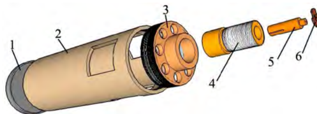
Рис. 2. Основні елементи піногенератора: 1) сітка 05 ГОСТ 3826; 2) стакан; 3) направляюча; 4) корпус; 5) розпилювач; 6) шайба
