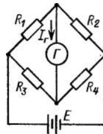
Рис. 2. Схема одинарного четырехплечевого моста постоянного тока
