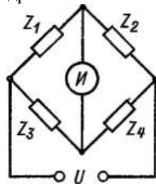
Рис. 1. Схема одинарного четырехплечевого моста
