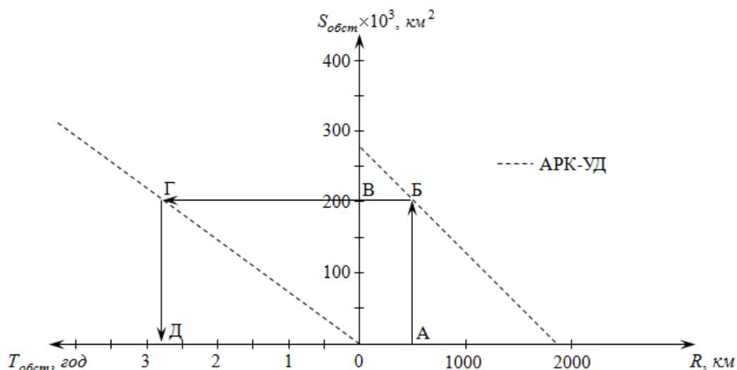
Рисунок 2— Графіки залежності площі обстеження ( S_{обст.} ) від часу обстеження ( T_{обст.} ) та радіусу польоту до району пошуку літака Ан-32П, обладнаного пристроєм радіотехнічного пошуку АРК-УД
