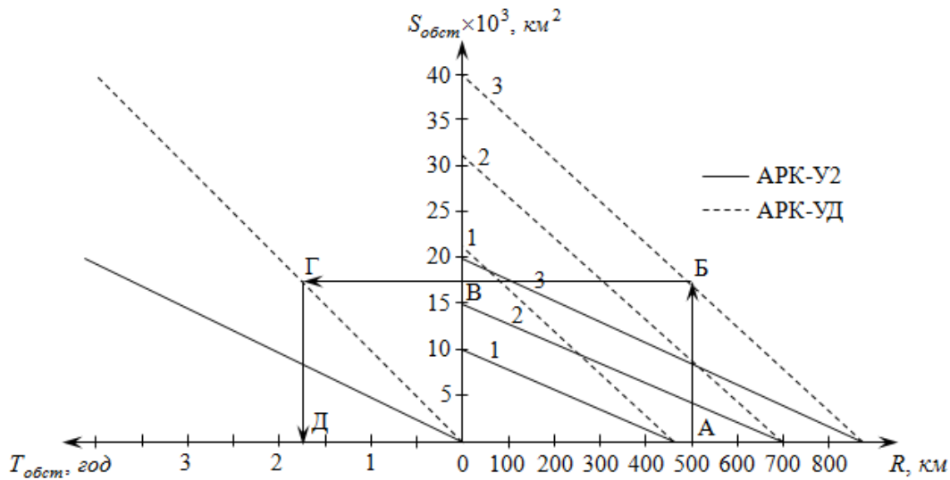
Рисунок 1– Графіки залежності площі обстеження ( S_{обст.} ) від часу обстеження ( T_{обст.} ) та радіуса польоту до району пошуку вертольоту Мі-8МТ, обладнаного пристроєм радіотехнічного пошуку АРК-У2 або АРК-УД при різних варіантах заправки паливом: 1 - G_T=1460 кг, 2 - G_T=2160 кг, 3 - G_T=2860 кг
