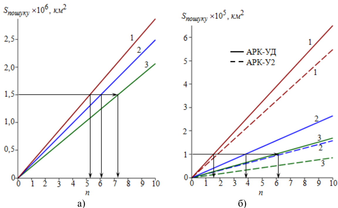
Рисунок 4 – Визначення мінімальної кількості однотипних повітряних засобів Ан-32П (а) або Мі-8МТ (б), необхідної для обстеження заданої площі пошуку при різних типах місцевості: 1 – поле, 2 – місто, 3 – ліс
