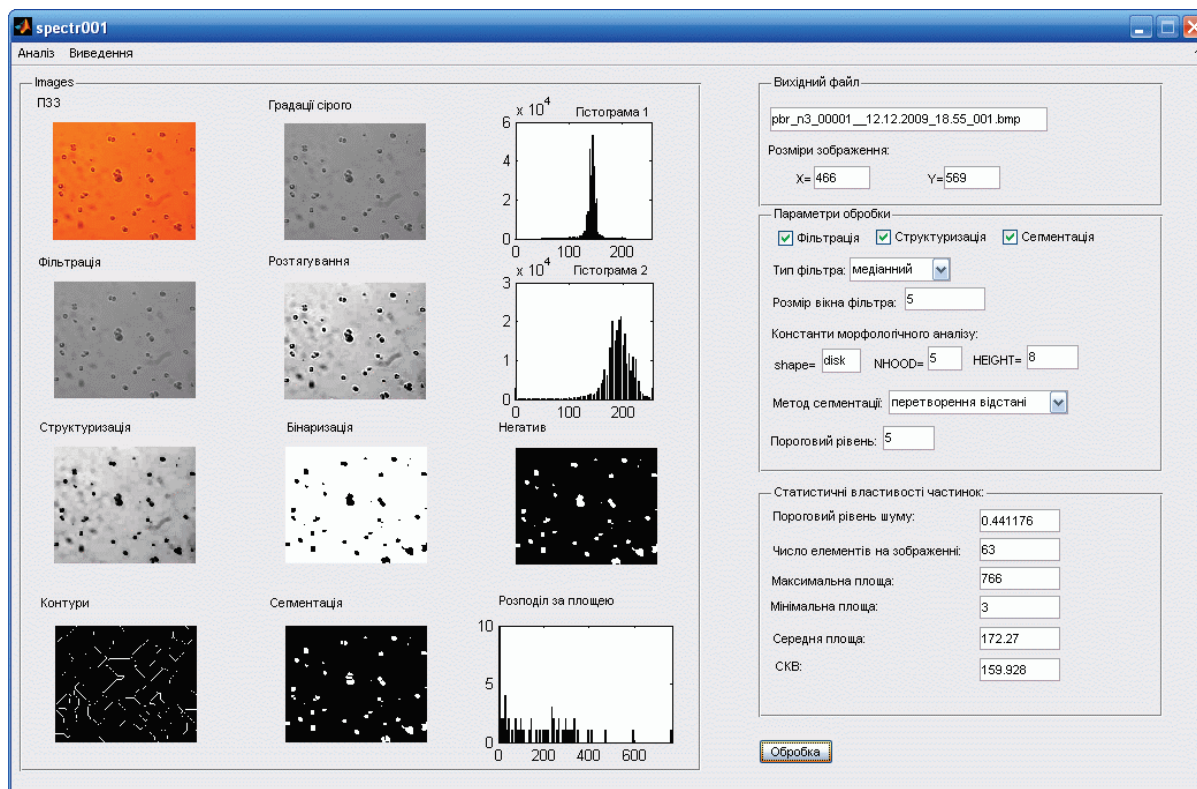
Рис. 1. Графічний інтерфейс користувача програми засобу контролю забруднення водних середовищ за спектрополяриметричним методом
