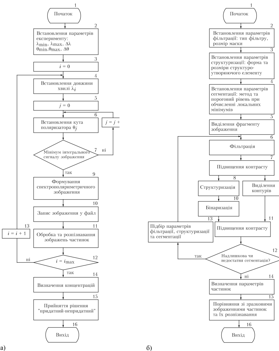
Рис. 2. Алгоритм роботи автоматизованого засобу контролю забруднення водних середовищ (а) і підпрограми обробки спектрополяриметричних зображень (б)
