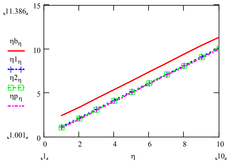
Рис. 1. Залежність співвідношень сигнал/шум на виході передавача \eta_k = h_{per}^2
