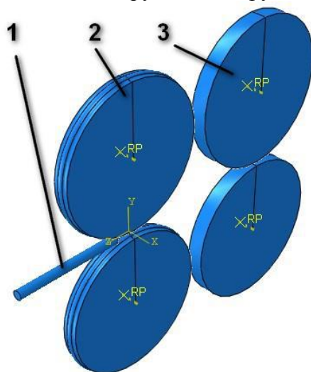
Рис. 2. Конечно-элементная в глобальной системе координат модель процесса плющения круглой проволоки (1 – заготовка; 2 – калибры с выпуклой бочкой первой клетки; 3 – валки с гладкой бочкой второй клетки)
