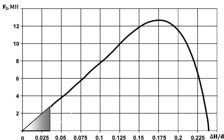
Рис. 3. Соотношение величин работы отрезки сдвигом и работы нанесения концентратора напряжений по способу «сдвиг–ломка»
