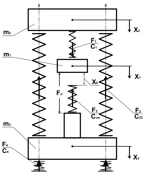
Рис. 2. Расчётная схема вертикального гидравлического пресса при мгновенном исчезновении технологической нагрузки
