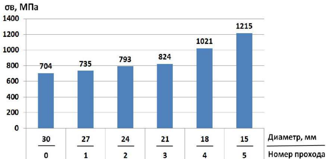
Рис. 4. Изменение предела прочности титана марки VT-1 после радиально-сдвиговой прокатки по проходам
