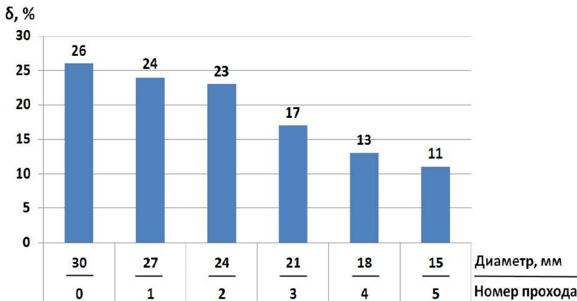
Рис. 5. Изменение относительного удлинения титана марки VT-1 после радиально-сдвиговой прокатки по проходам
