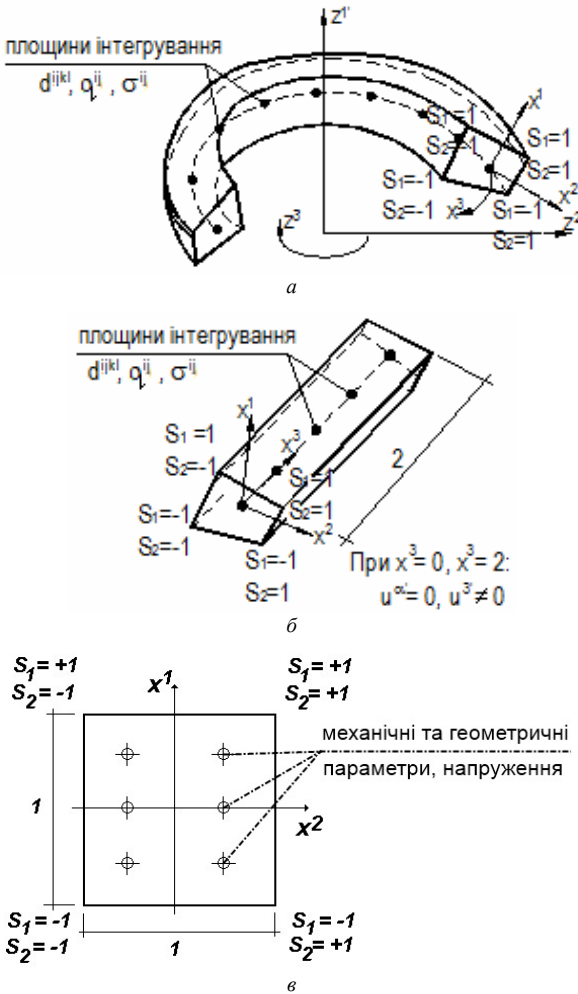
Рис. 1. Скінченні елементи на основі рядів Фур'є: а) замкнутий круговий; б) шарнірно опертий призматичний; в) точки інтегрування у площині
