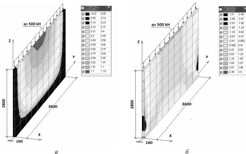
Рис. 4. Ізолінії згинальних моментів M_{x3} , \text{кНм} :
