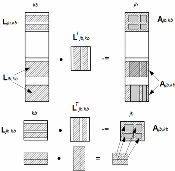
Рис. 2. Поправка блок-столбца jb блок-столбцом kb , расположенным слева. Нулевые строки в блоках заштрихованы. Серым цветом показаны поправляемые подблоки в блок-строке jb . Внизу показан пример упаковки при умножении блоков
