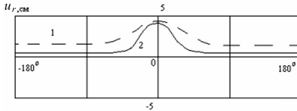
Рис. 9. Переміщення серединної поверхні каркасу у радіальному напрямку по стінці: 1 – результати [24], 2 – МСЕ рішення
