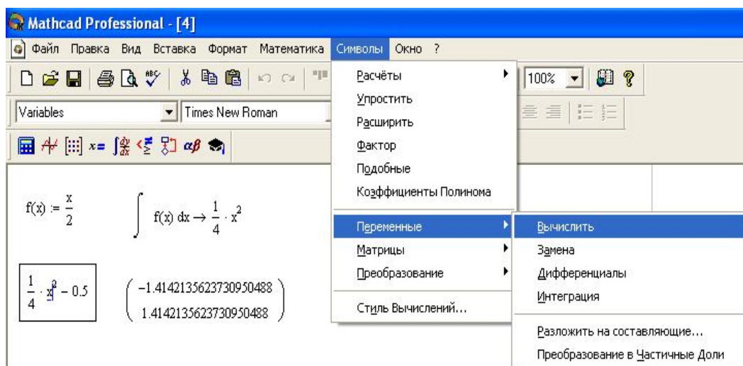
Рис. 11. Обчислення медіани
