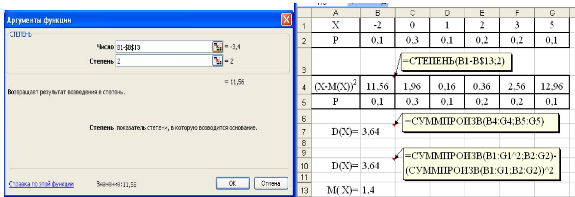
Рис. 2. Обчислення дисперсії
