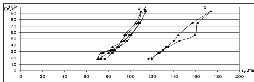
Рис. 1. Реограми гелів з бодягою на основі «Aristoflex AVC», де: 1 – свіжо приготований зразок; 2 – зразок через 1 рік; 3 – зразок через 2 роки.
