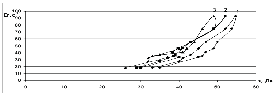
Рис. 1. Реограми гелів з бодягою на основі «Aristoflex AVC», де: 1 – свіжо приготований зразок; 2 – зразок через 1 рік; 3 – зразок через 2 роки.
