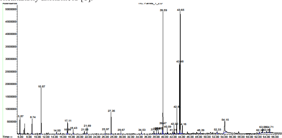
Рис. 2. Хроматограма ГХ-МС-аналізу метилових ефірів летких компонентів стевії
