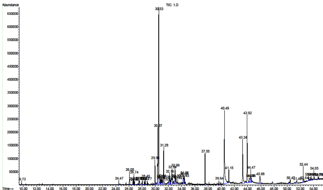
Рис. 1 Хроматограма ГХ-МС-аналізу леткої фракції стевії, одержаної методом перегонки із водяною парою
