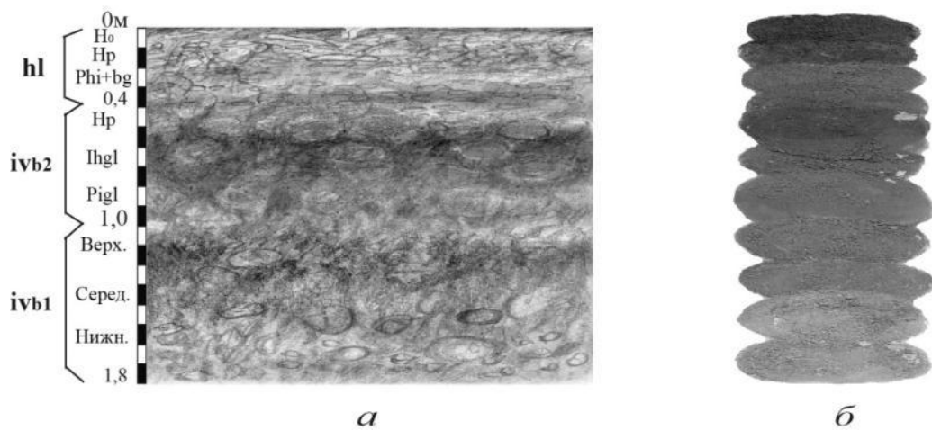
Рис.5. Місцезнаходження Великий Шолес. Зачистка №2: I – вид з півдня (фото); II – польова зарисовка (a) і примазки природного матеріалу (б)
