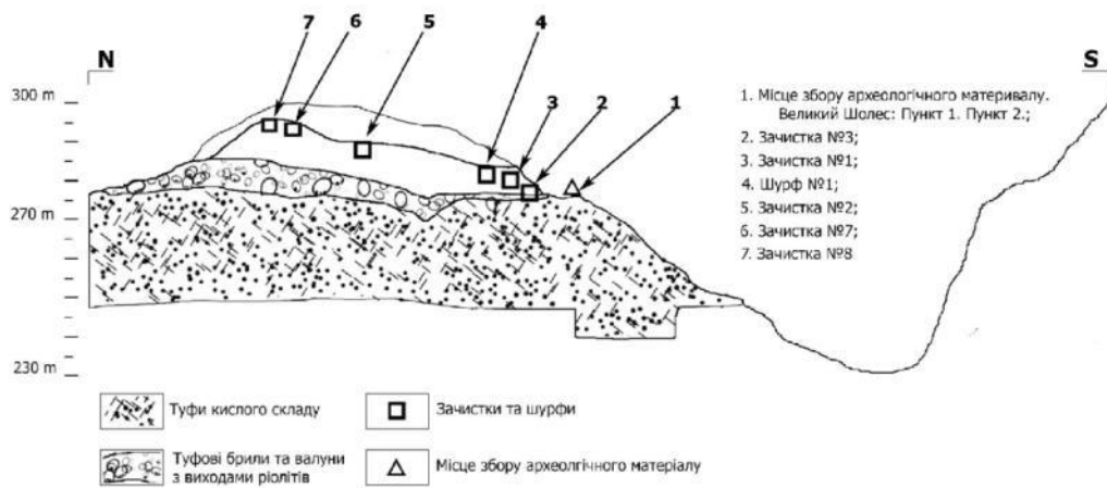
Рис. 3. Схематичний геологічний профіль Великокораковецького туфового кар'єру. Розташування основних об'єктів дослідження на місцезнаходженні Великий Шолес
