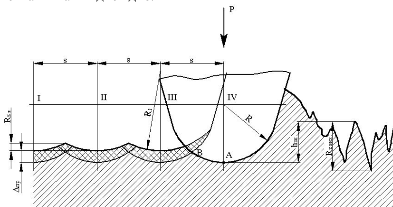
Рис. 2. Схема для розрахунку висоти мікронерівностей при вигладжуванні
