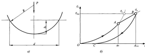
Рис. 1. Рух металу при втискуванні сферичного вигладжувача
