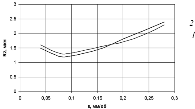
Рис. 3. Залежність шорсткості поверхні Rz від подачі s при вигладжуванні (1 - сталь ШХ15, P=100H , R=1,5mm ; 2 - сталь ШХ15, P=250H , R=1,5mm )
