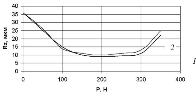
Рис. 4. Вплив сили вигладжування на шорсткість поверхні (1 – R_v = 1,5\text{мм} , сталь ШХ15, n=650\text{об/хв} , s=0,08\text{мм} ; 2 - R_v = 1,5\text{мм} , сталь ШХ15, n=650\text{об/хв} , s=0,12\text{мм} )
