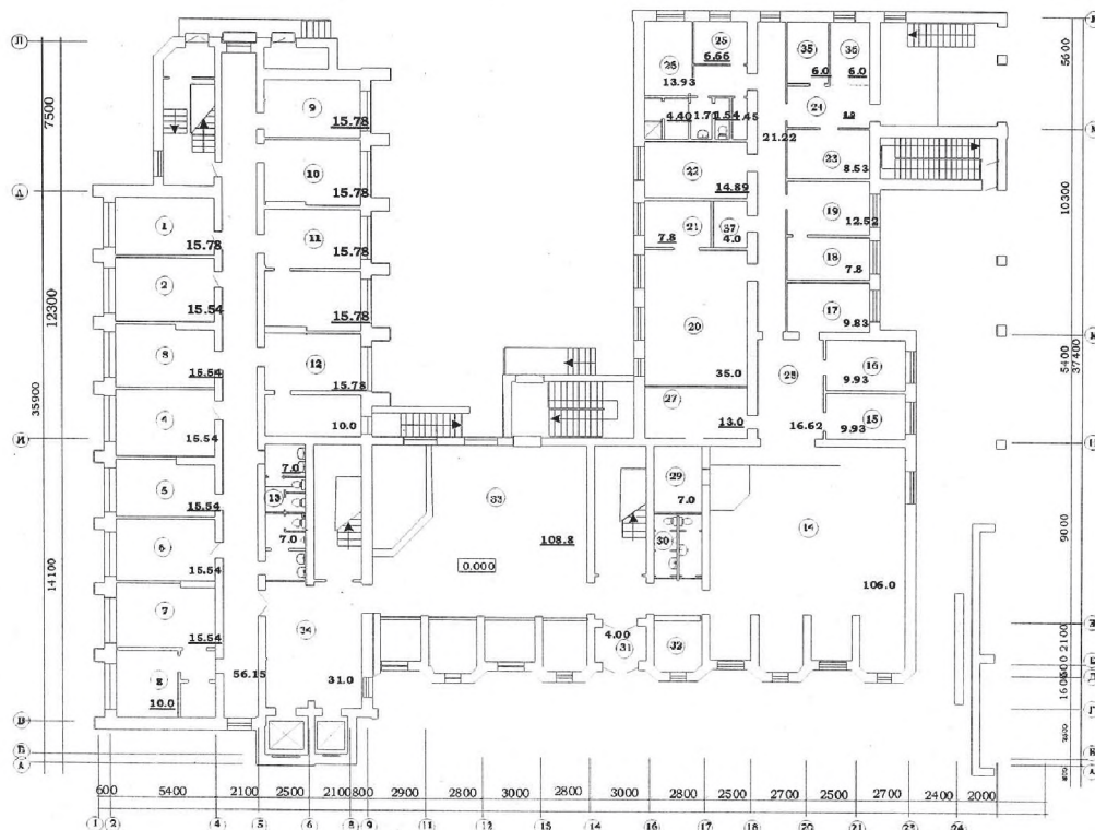
План 1 этажа
