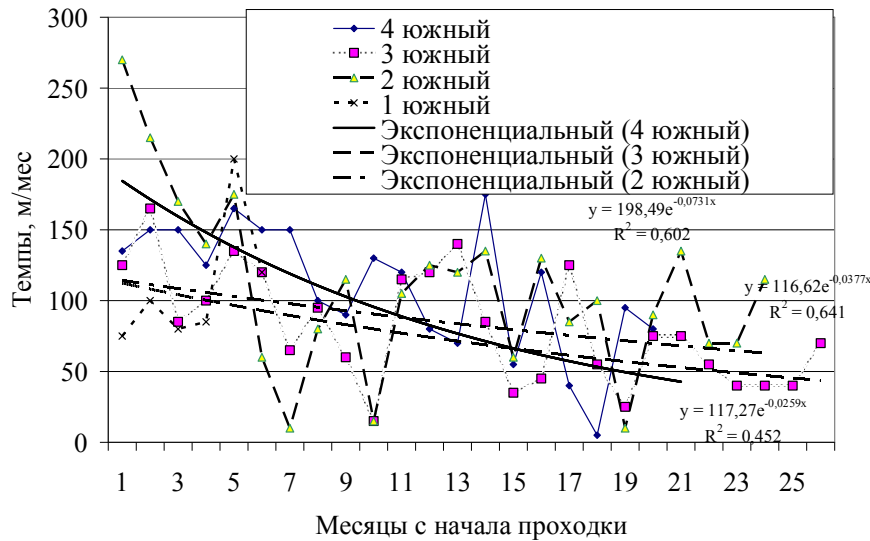
Рис. 1. Характер изменения темпов проходки с удлинением выработки при неизменной технологии и условий проведения
