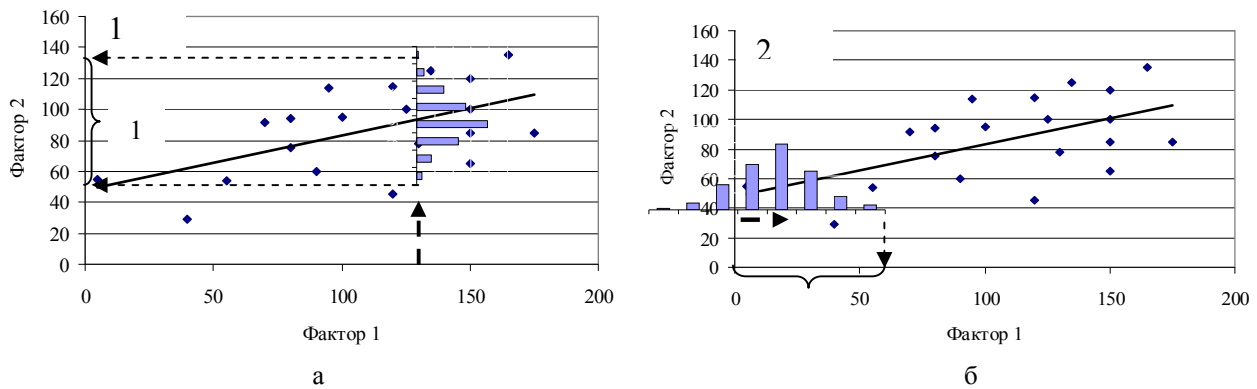
Рис. 3. Техника са́мплинга с учетом корреляции между входными факторами
